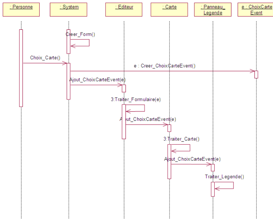
Figure 4.10 : La gestion événementielle en cascade de la version 0.9
