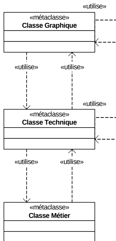
Figure 5.1 : Diagramme de classes de l'architecture logicielle
