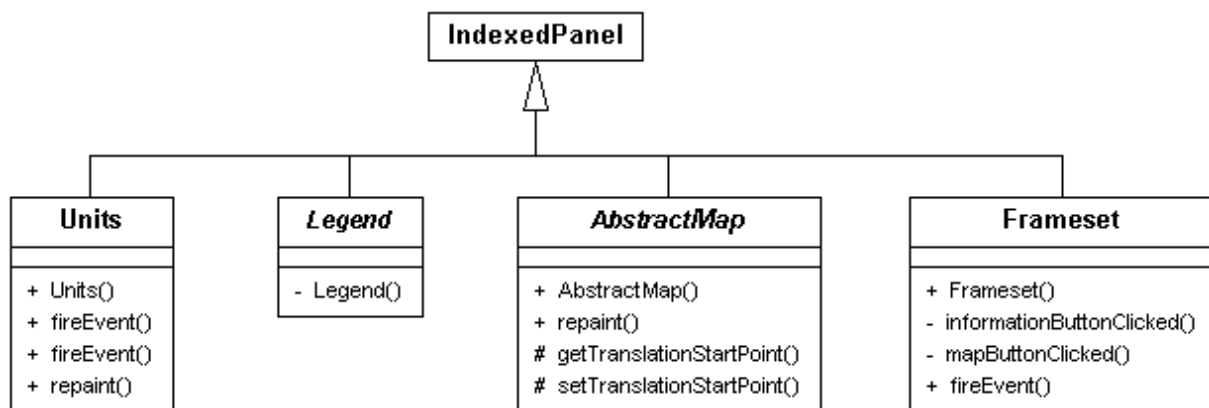
Figure 5.8 : Diagramme de classes : abstraction de la classe IndexedPanel
