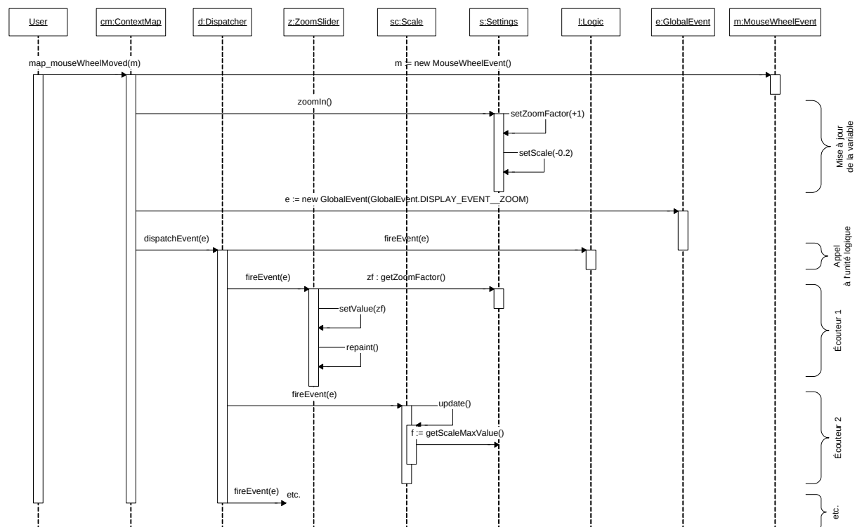
Figure 5.7 : Diagramme de séquence : zoom avant par la molette de la souris de l'utilisateur
