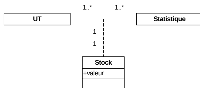
Figure 3.7 : Diagramme de classes : UT et statistiques
