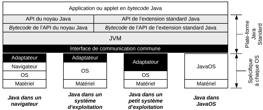
Figure 2.4 : La plate-forme Java est identique sur tous les OS, d'après [KRAM, 96]
