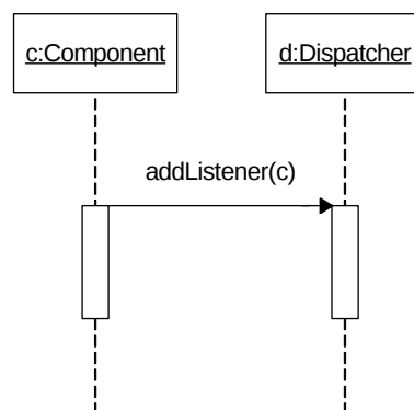
Figure 5.3 : Diagramme de séquences : enregistrement d’un écouteur
