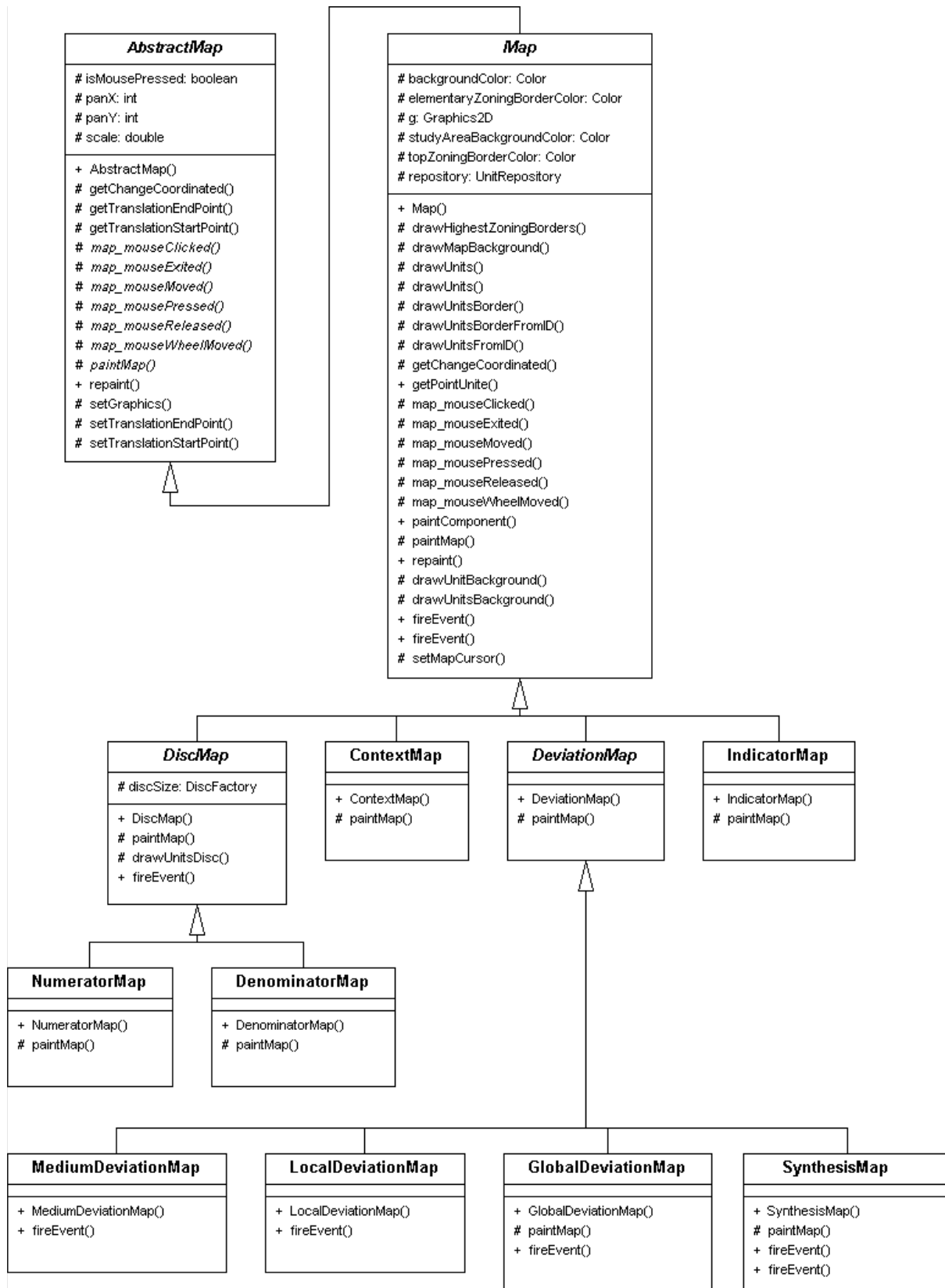
Figure 5.9 : Diagramme de classes : héritage des classes de carte
