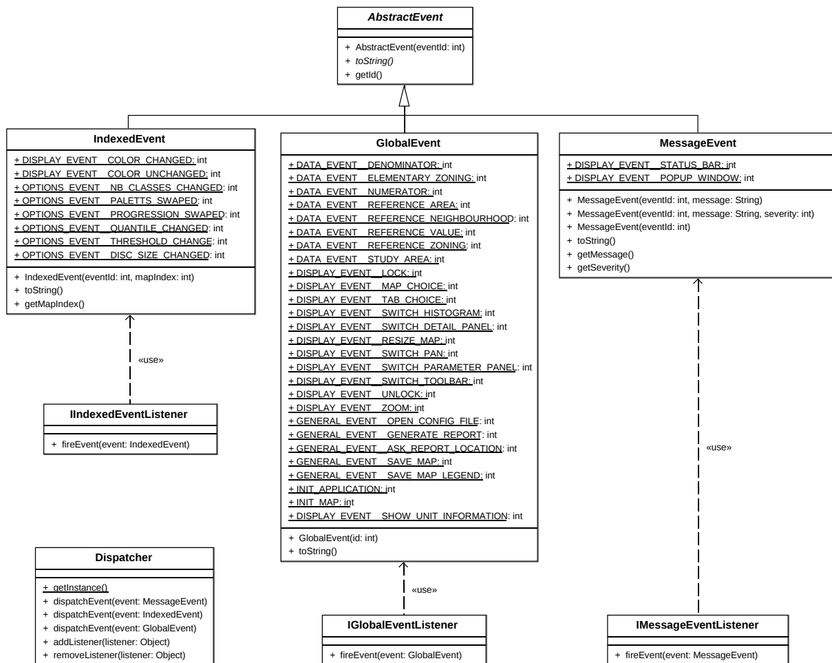
Figure 5.2 : Diagramme des classes et des interfaces implémentant le principe de dispatcher d'événements
