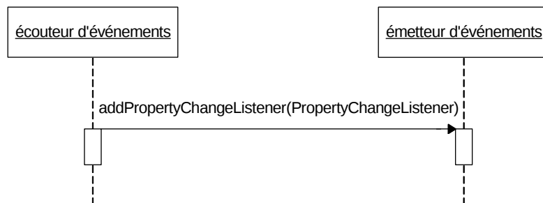
Figure 4.8 : Enregistrement d’un écouteur auprès d’un composant émetteur d’événements
