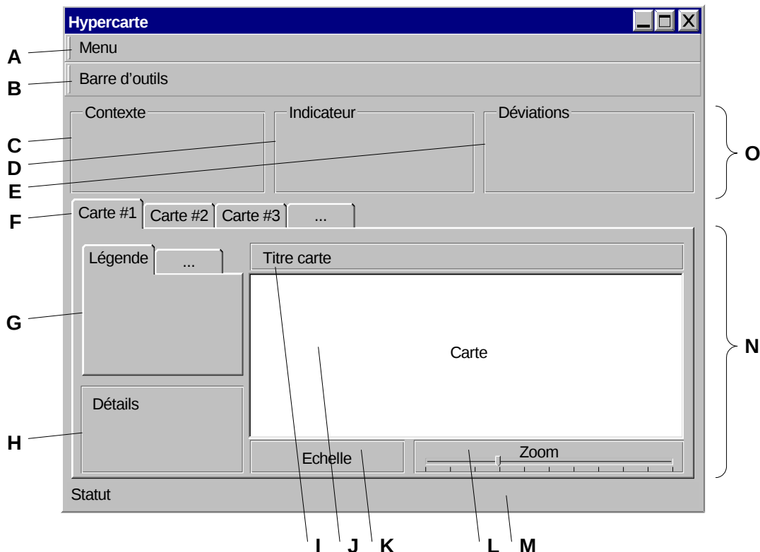
Figure 6.4 : Structure de l'interface de la version 1.0
