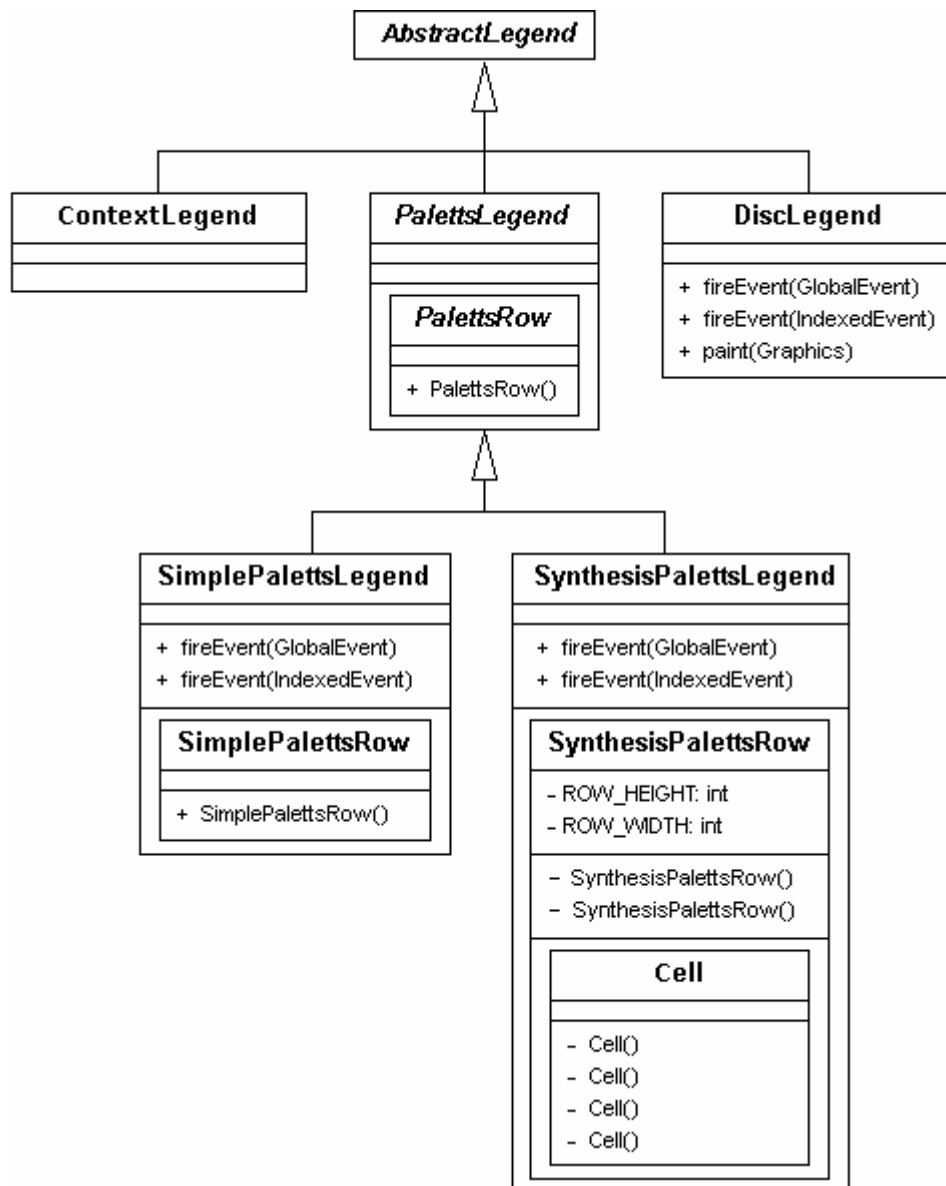
Figure 5.10 : Diagramme de classes : héritage des classes de légendes
