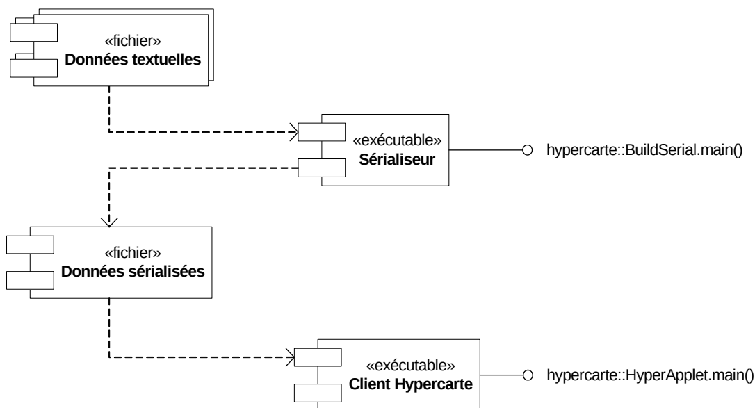
Figure 4.1 : Diagramme de composants : les composants d'Hypercarte (vue macroscopique)
