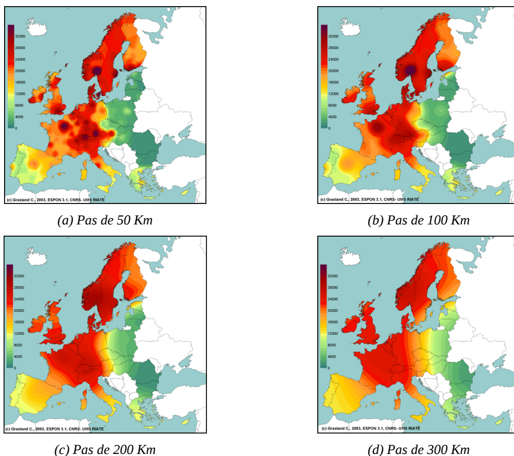
Figure 7.2 : Distribution lissée du PIB par habitant à différents pas de voisinage gaussien, d'après [GRAS, 04]
