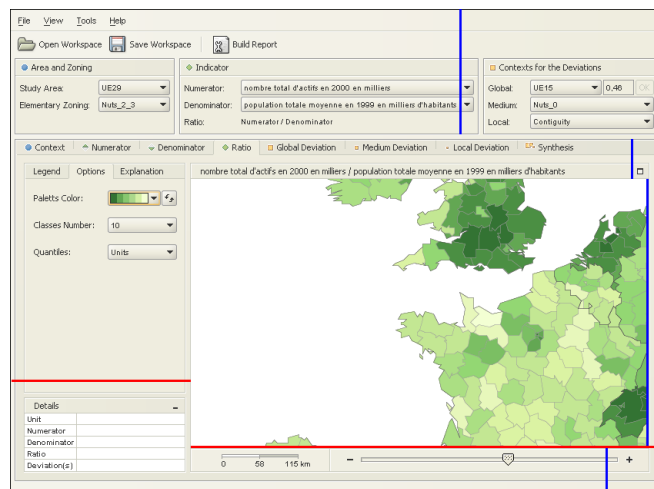
Figure 6.13 : Axes de redimensionnement dynamiquement au changement de taille de fenêtre de l'interface de la version 1.0
