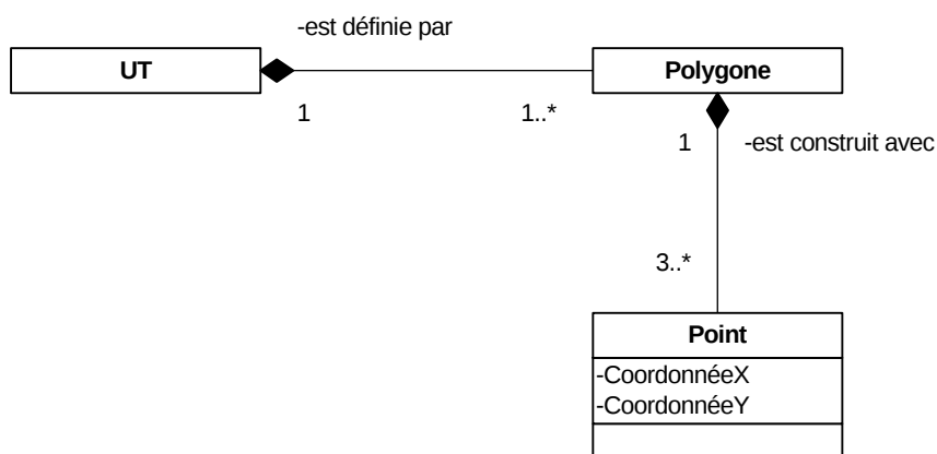
Figure 3.8 : Diagramme de classes : UT et géométrie
