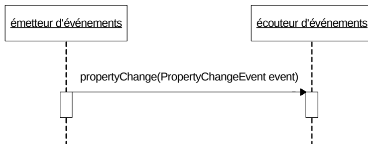
Figure 4.9 : Signalement d’un évènement à l’écouteur par le composant émetteur d’événements
