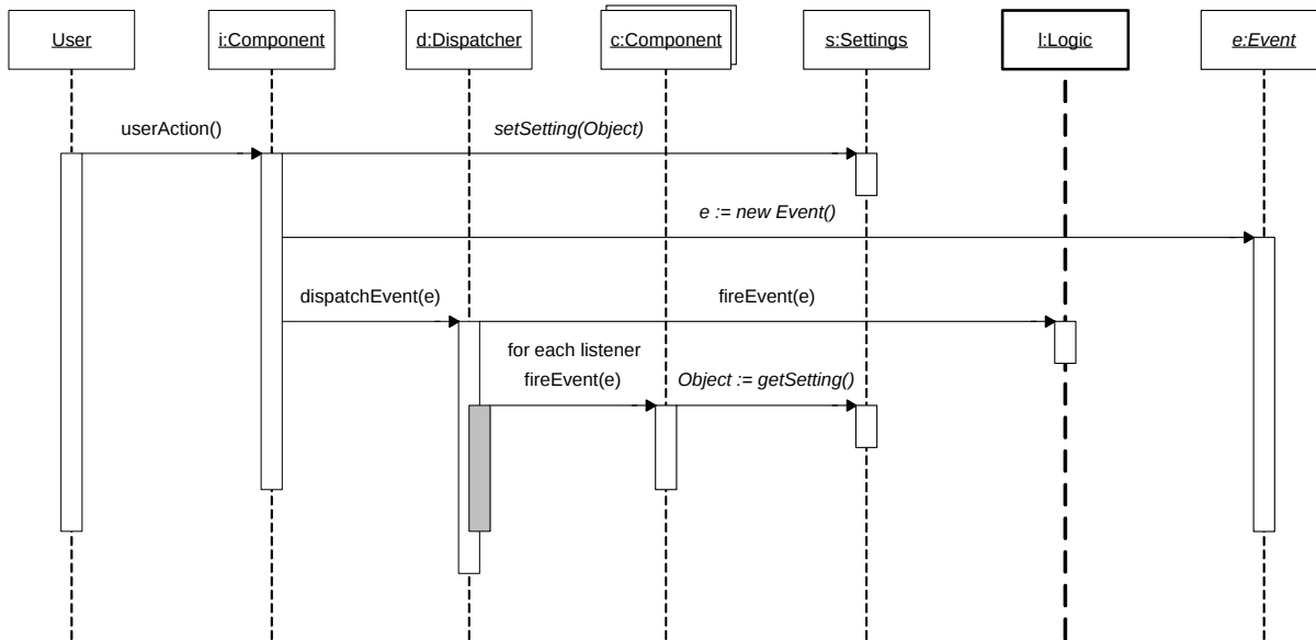
Figure 5.6 : Diagramme de séquences : intégration de la logique métier
