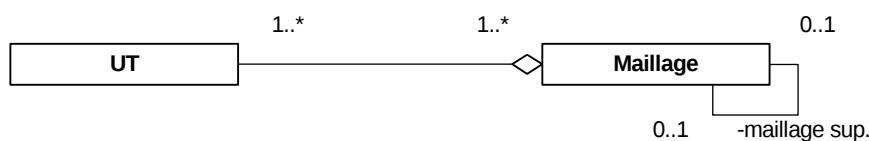
Figure 3.4 : Diagramme de classes : unités territoriales et maillages
