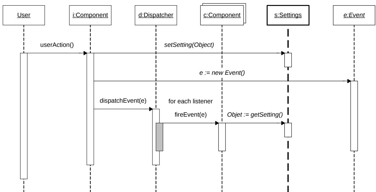
Figure 5.5 : Diagramme de séquences : intégration de la classe Settings
