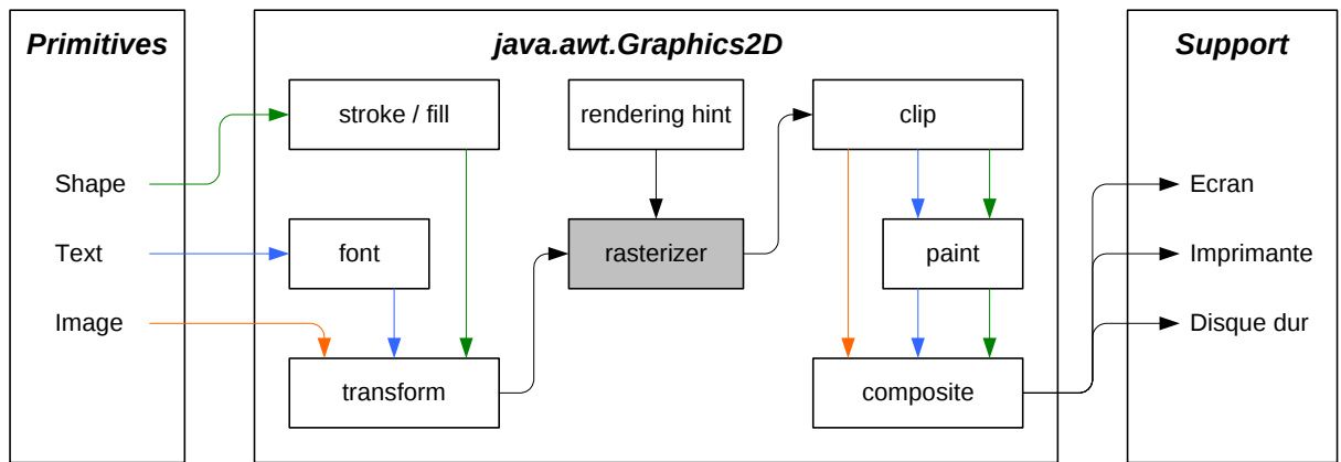
Figure 2.5 : Enchaînement des tâches lors du processus de rendu effectué par la classe java.awt.Graphics2D
