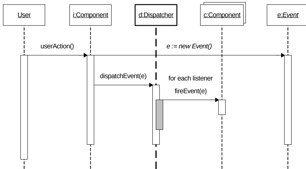
Figure 5.4 : Diagramme de séquence : propagation d'un événement
