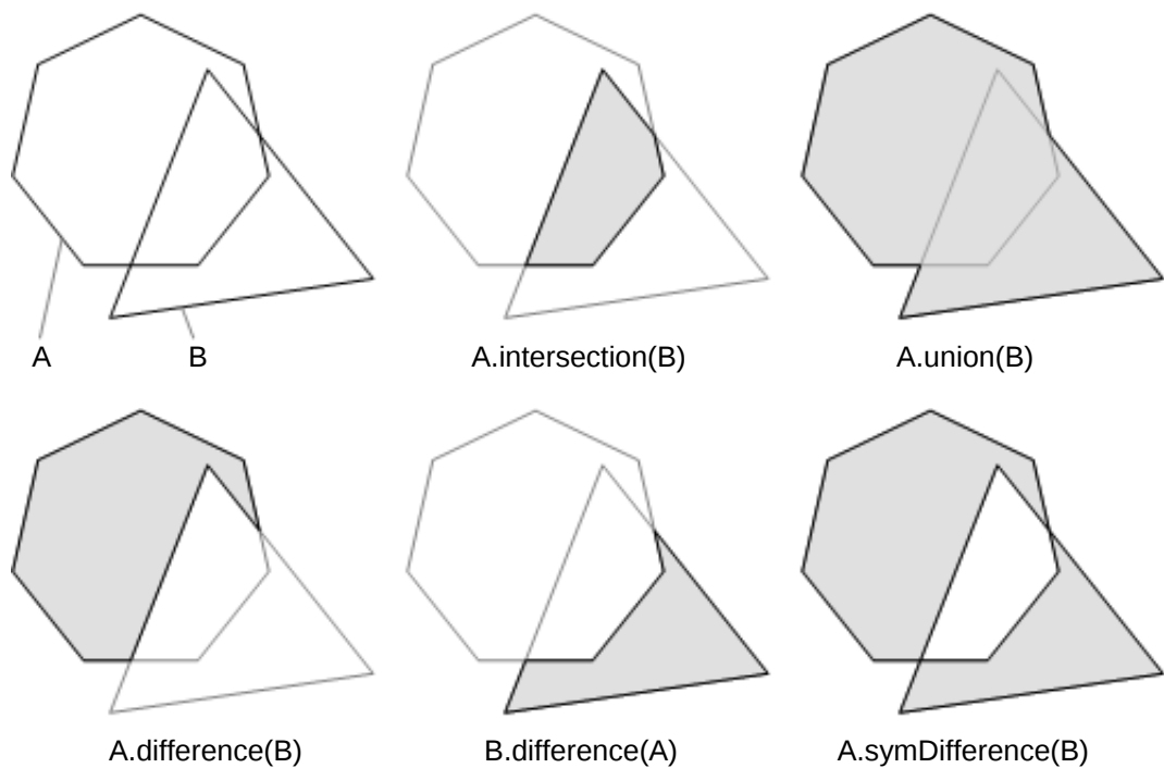
Figure 2.6 : Les opérations géométriques possibles avec JTS
