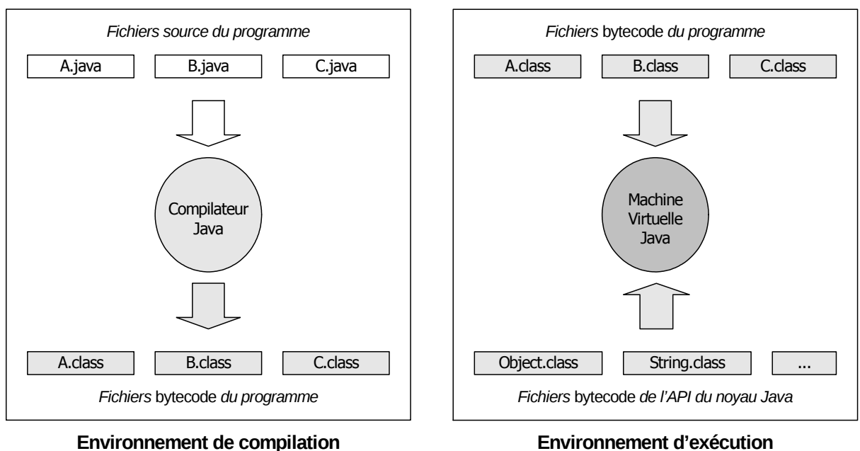
Figure 2.3 : Principes de fonctionnement de Java : compilation et exécution
