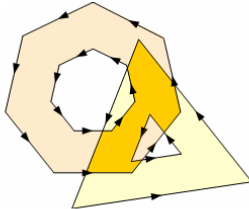
Figure 2.7 : La technique des chaînes monotones utilisée par JTS appliquée ici à l'intersection de deux polygones troués
